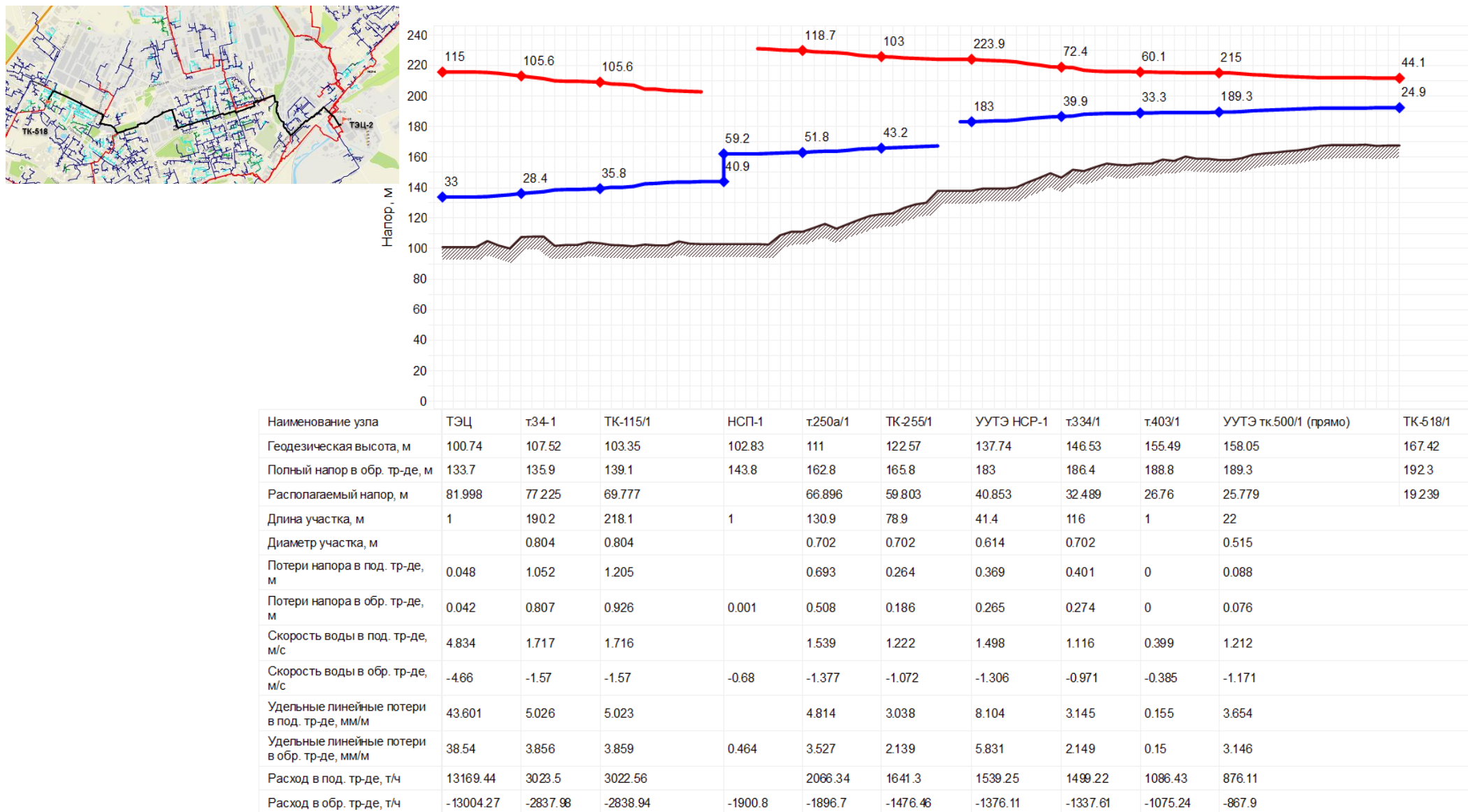
Рисунок 10 – Пьезометрический путь от ТЭЦ-2 до наиболее отдалённой контрольной камеры ТК-518 (7,4 км)
